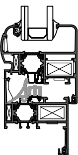
Anta Linea Tonda infilare
