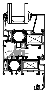
Telaio complanare
