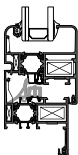
Anta Linea Curva Vetro infilare
