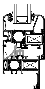
Anta Linea Curva
