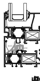
Telaio complanare arrotondato
