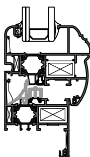
Anta Linea Curva-Scorniciata Vetro infilare
