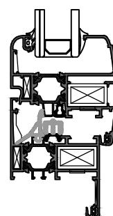
Anta Linea Curva-Arrotondata Vetro infilare
