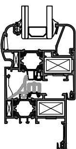
Anta Linea Tonda
