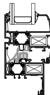
Anta Linea Retta-Arrotondata Vetro infilare
