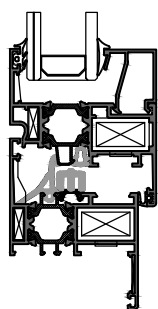
Telaio sormonto
