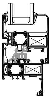
Anta Linea Retta Vetro infilare
