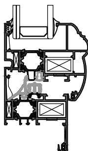
Anta Linea Retta-Scorniciata Vetro infilare
