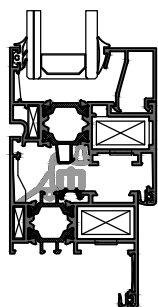
Anta Linea Retta
